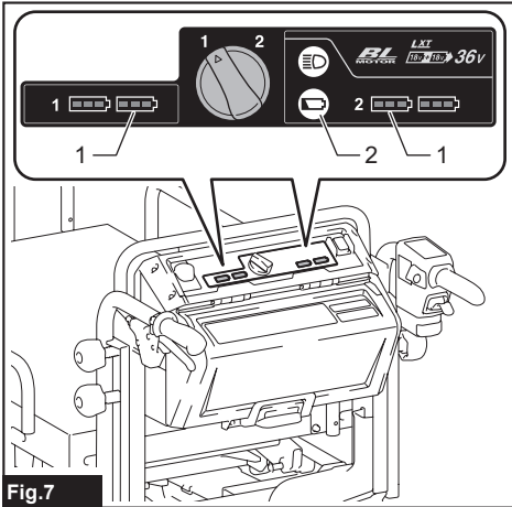
Fig.7 1. Indicador de batería 2. Botón de verificación
