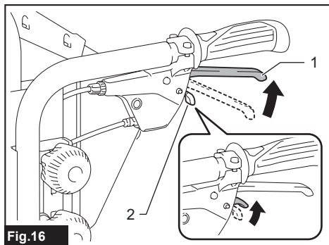
► 1. Palanca del freno 2. Palanca de bloqueo
